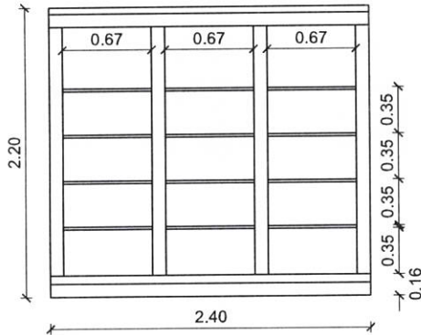
MUEBLE B1
