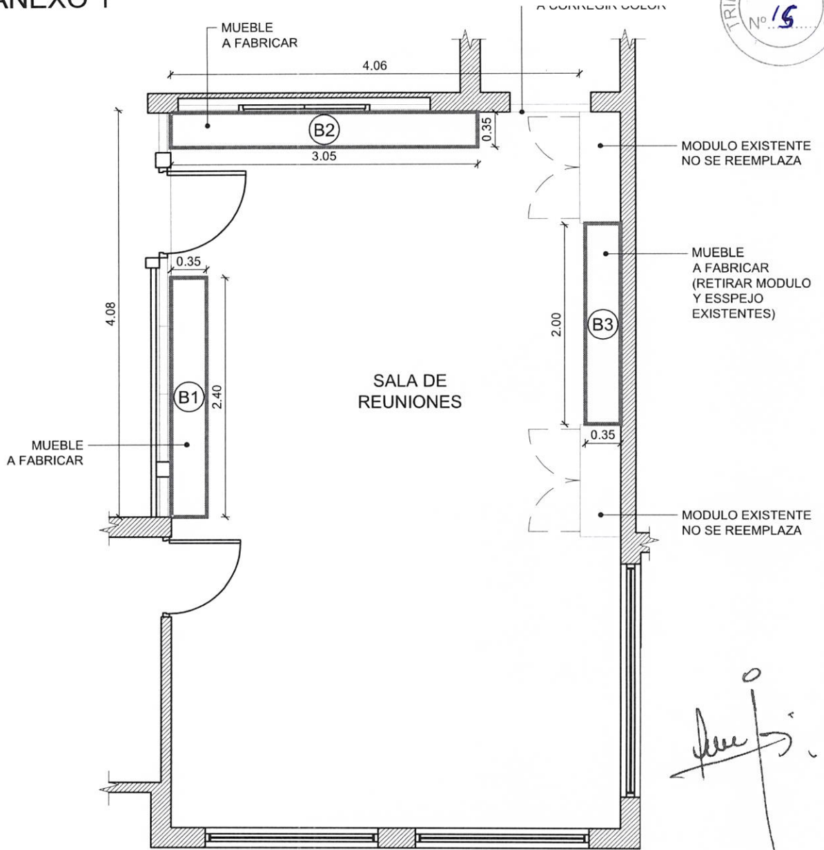
PLANTA BAJA
